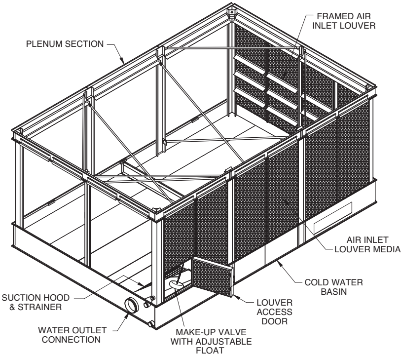
PAN & PLENUM SECTION
