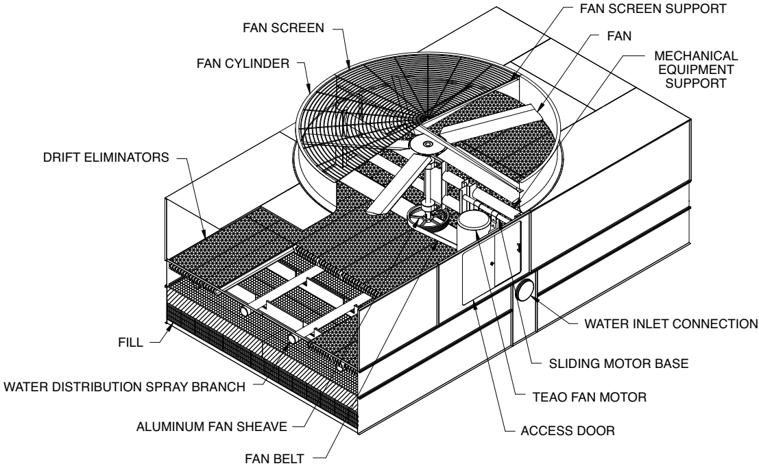
FAN & FILL CASING SECTION
