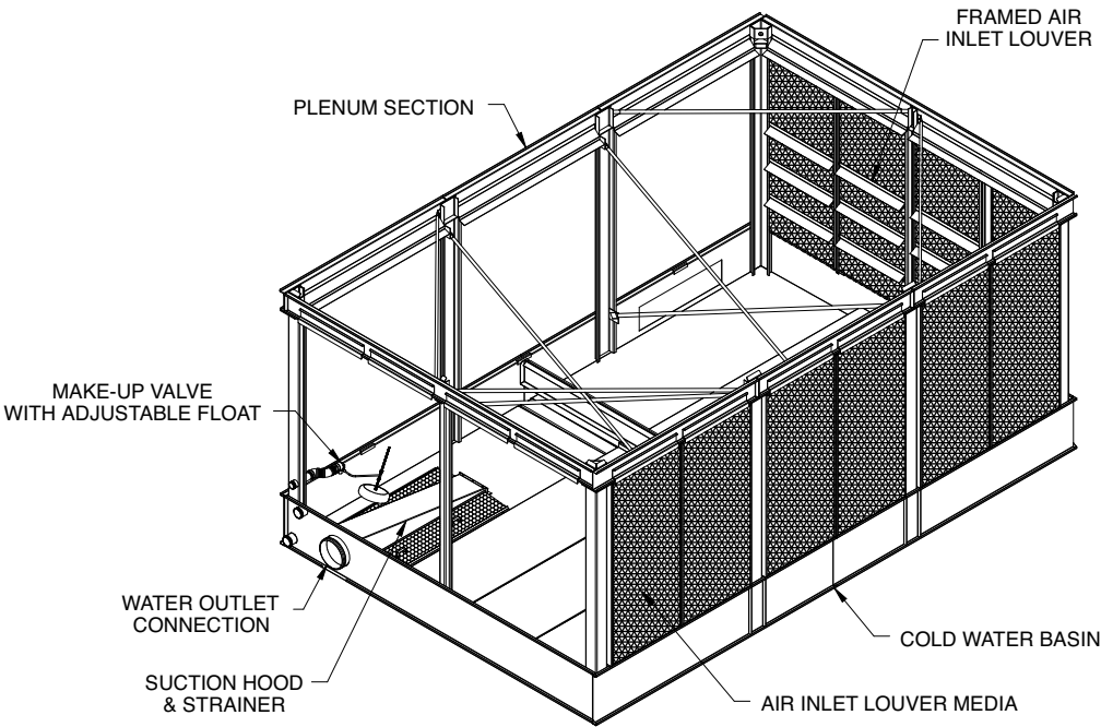
PAN & PLENUM SECTION
