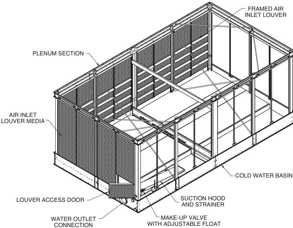
PAN & PLENUM SECTION
