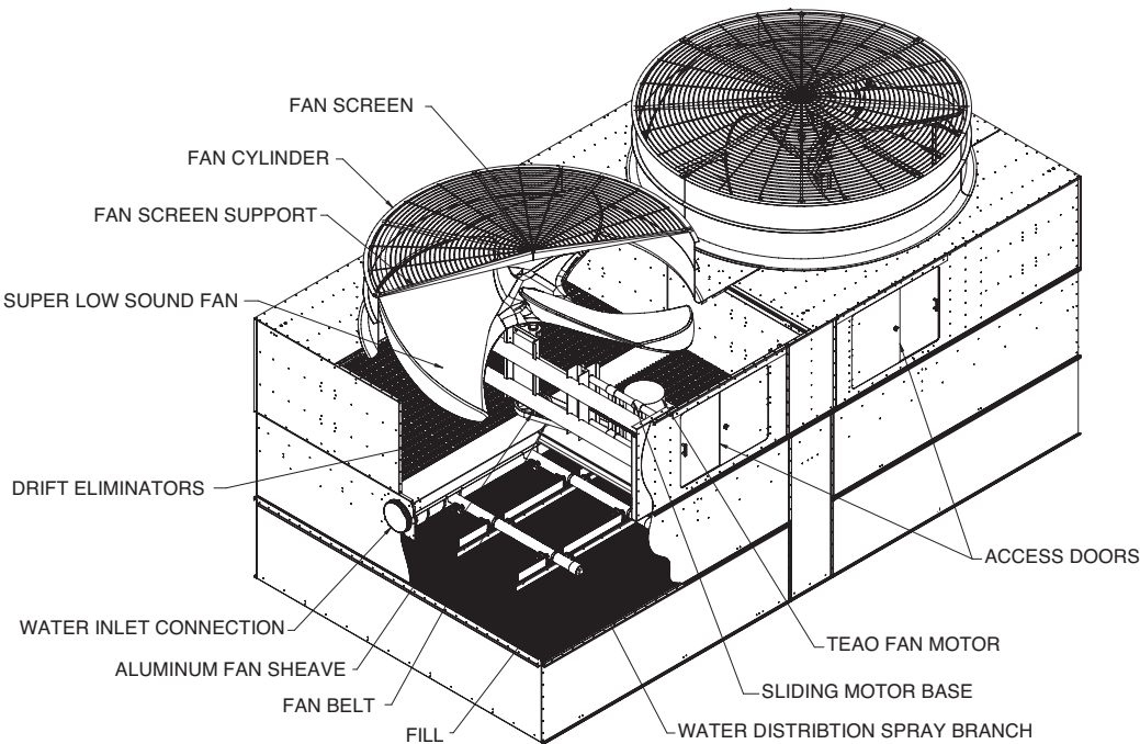
FAN & FILL CASING SECTION
